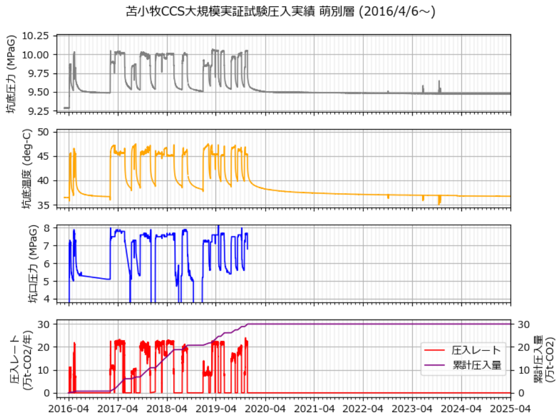
図 3.1-1 萌別層圧入井の圧入履歴
