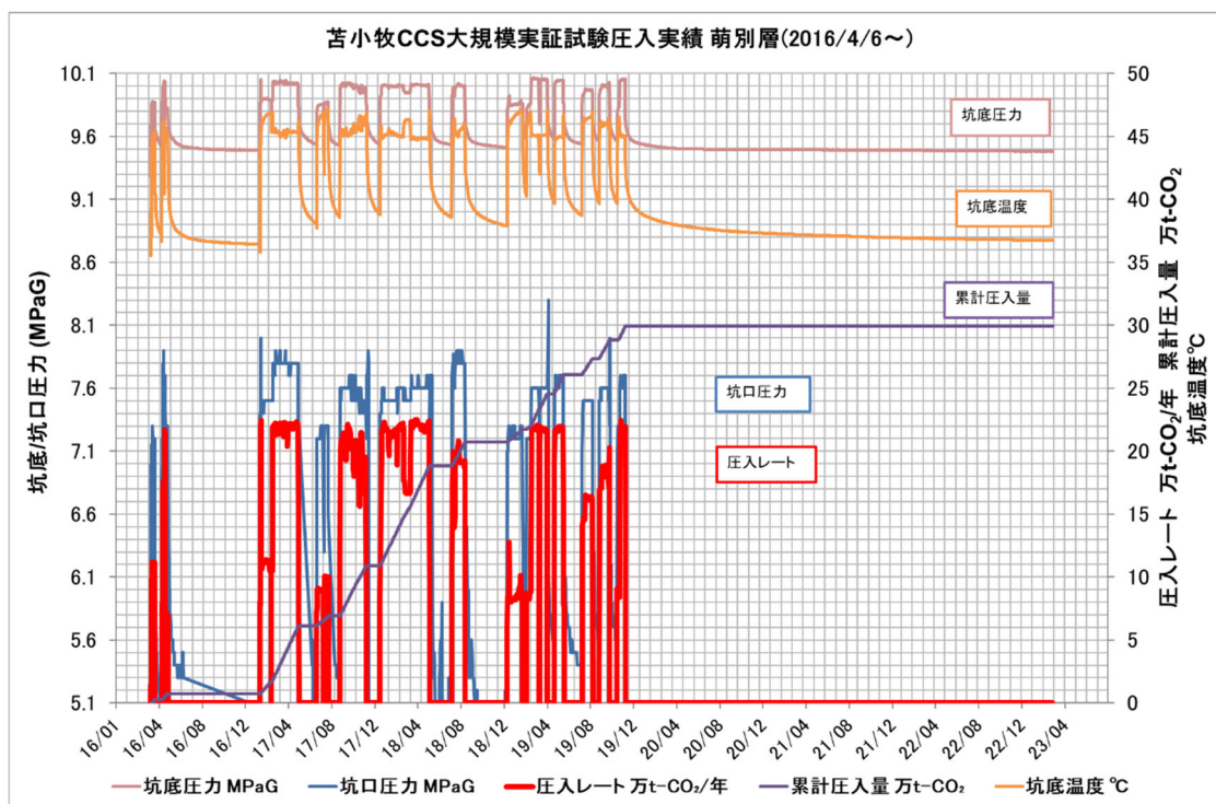
図 3.1-1 萌別層圧入井の圧入履歴
