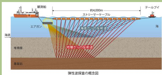
弾性波探査の概念図
